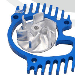
SM Project - Kit bomba água maior volume TM 250-300 2T >2019 SM_039
